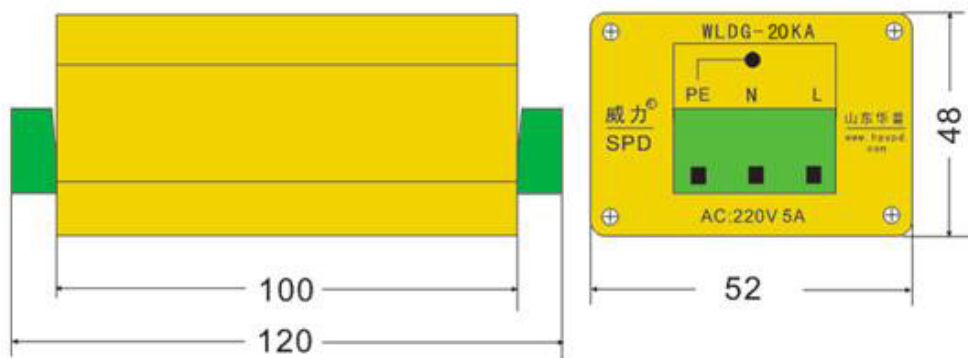
小功率电源SPD安装尺寸
